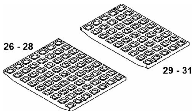
Abbildung 4: Modulare Regalauflagen
