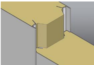
TectoCell Standard Plus überlappende Wände ohne Fugen gegen Staub und Bakterien
