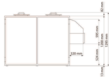
Nassmüllkühler 2 x 240 l
