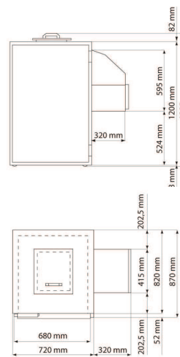
Nassmüllkühler 2 x 240 l
