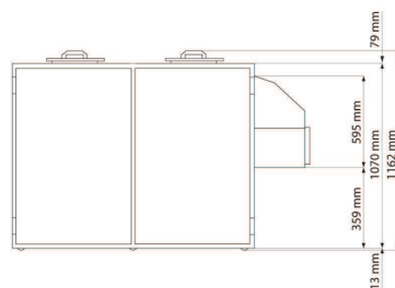
Nassmüllkühler 2 x 120 l
