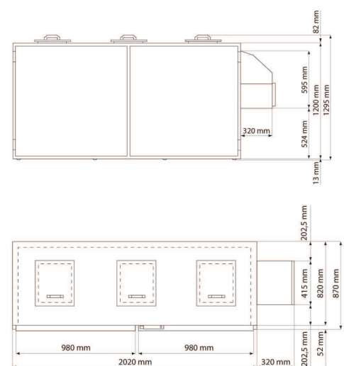
Nassmüllkühler 3 x 240 l °C +4.+20
