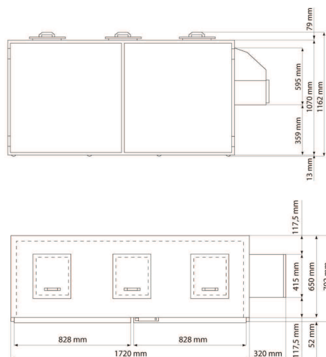
Nassmüllkühler 3 x 120 l °C +4.+20
