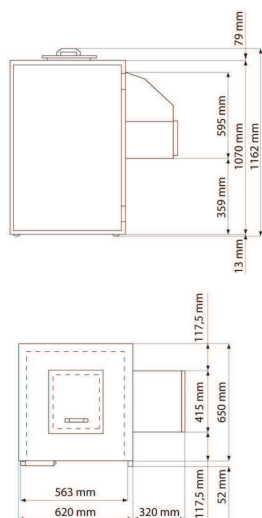
Nassmüllkühler 2 x 120 l
